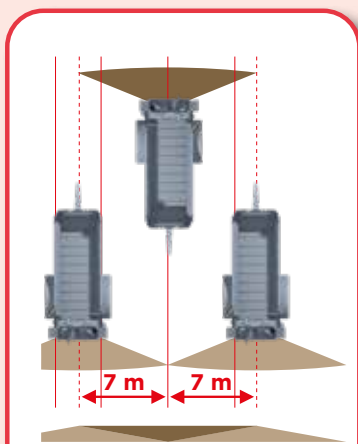
Kruisingsbreedtes (variabel afhankelijk van het gestrooide materiaal) 7 m (standaard) of 8 m met afgeronde messen.
