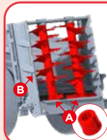
(A) Verwisselbare slijtringen (behalve op 37S08 en 42S09). (B) Gecentraliseerde smeerpunten op de strooiwalsen.
